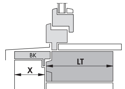
III. C – canal d'allège (BK) (4)
