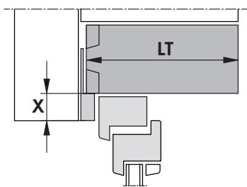
Fig. B: piastrina a vista, canalina stipite/architrave (4)
