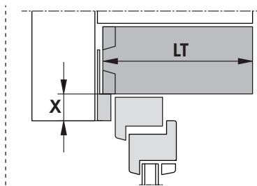
III. B – plaque de finition, canal d'ébrasement / de linteau (4)
