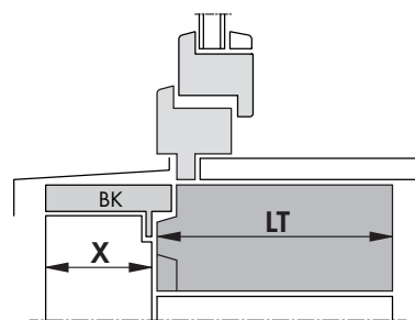
III. C – canal d'allège (BK) (4)
