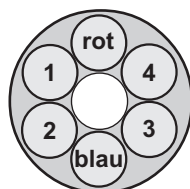
Anschlusskabel
