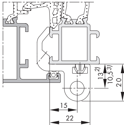
Point de rotation LM 4200 / 3100
