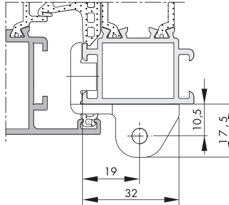
Point de rotation LM PC/TRAP.
