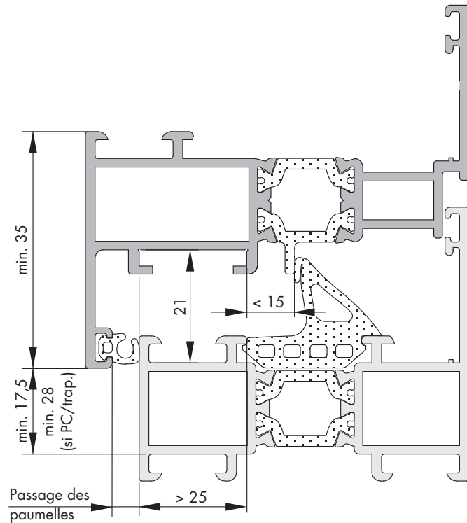
Point de rotation LM 4200 / 3100
